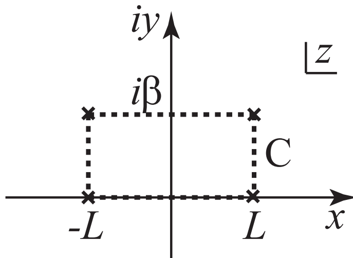
図 7.3 積分経路
