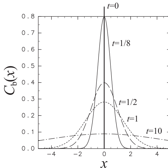
図 7.2 基本解 C_b(x) の発展. 太実線 ( t = 0 ), 細実線 ( t = 1/8 ), 破線 ( t = 1/2 ), 点線 ( t = 1 ), 一点鎖線 ( t = 10 ). \kappa の値は 1 とした.
