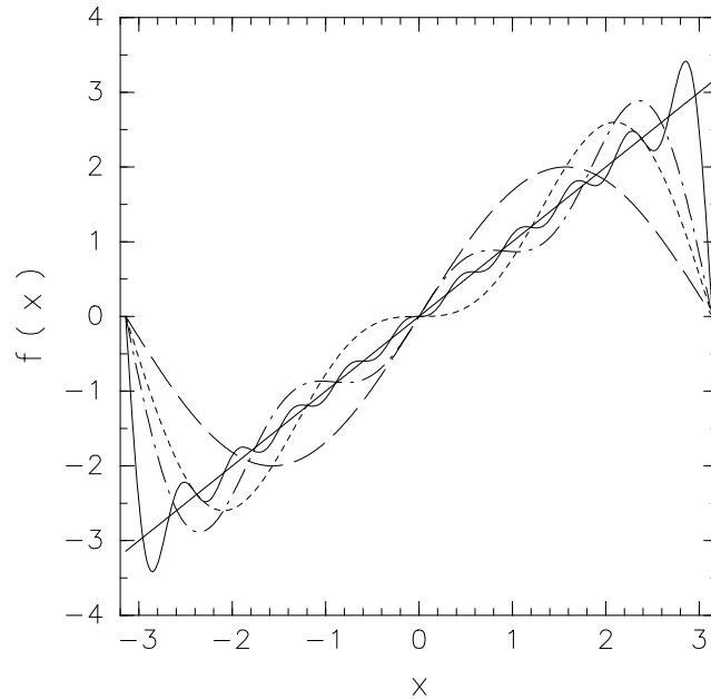
図 2.1 太実線は f(x) = x . 破線は f(x) の Fourier 級数展開の初項を, 点線は f(x) の Fourier 級数展開の第 2 項まで, 一点破線は f(x) の Fourier 級数展開の第 3 項まで, 細実線は f(x) の Fourier 級数展開の第 10 項目までを图示した.
