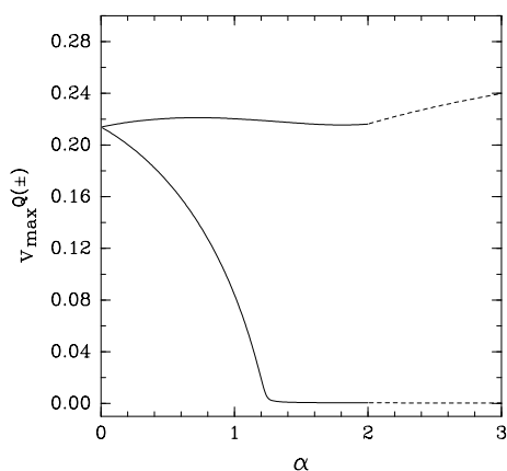
図2 局所性関数 L_{\alpha}^{\mathcal{Q}(\pm)}(v) が最大となる波数比 v_{\max}^{\mathcal{Q}(\pm)} の \alpha 依存性. 太線は v_{\max}^{\mathcal{Q}(+)} を, 細線は v_{\max}^{\mathcal{Q}(-)} を表す. 図1と同様に \alpha > 2 ではエンストロフィースペクトルのスケーリング則の導出に失敗しているので, 参考のために点線で記している.
