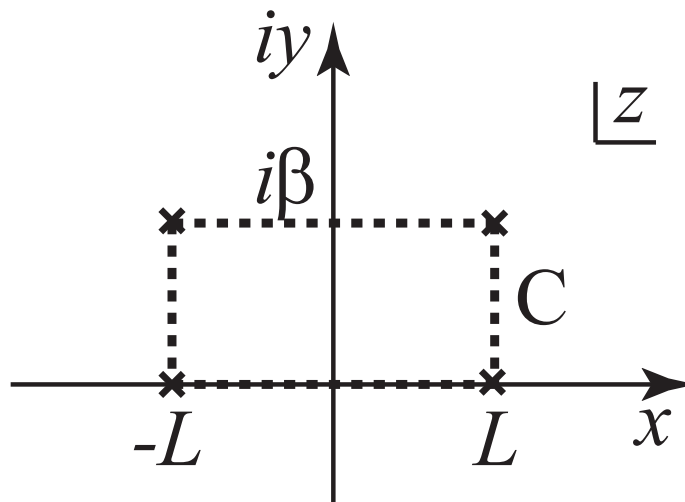
図 6.3 積分経路
